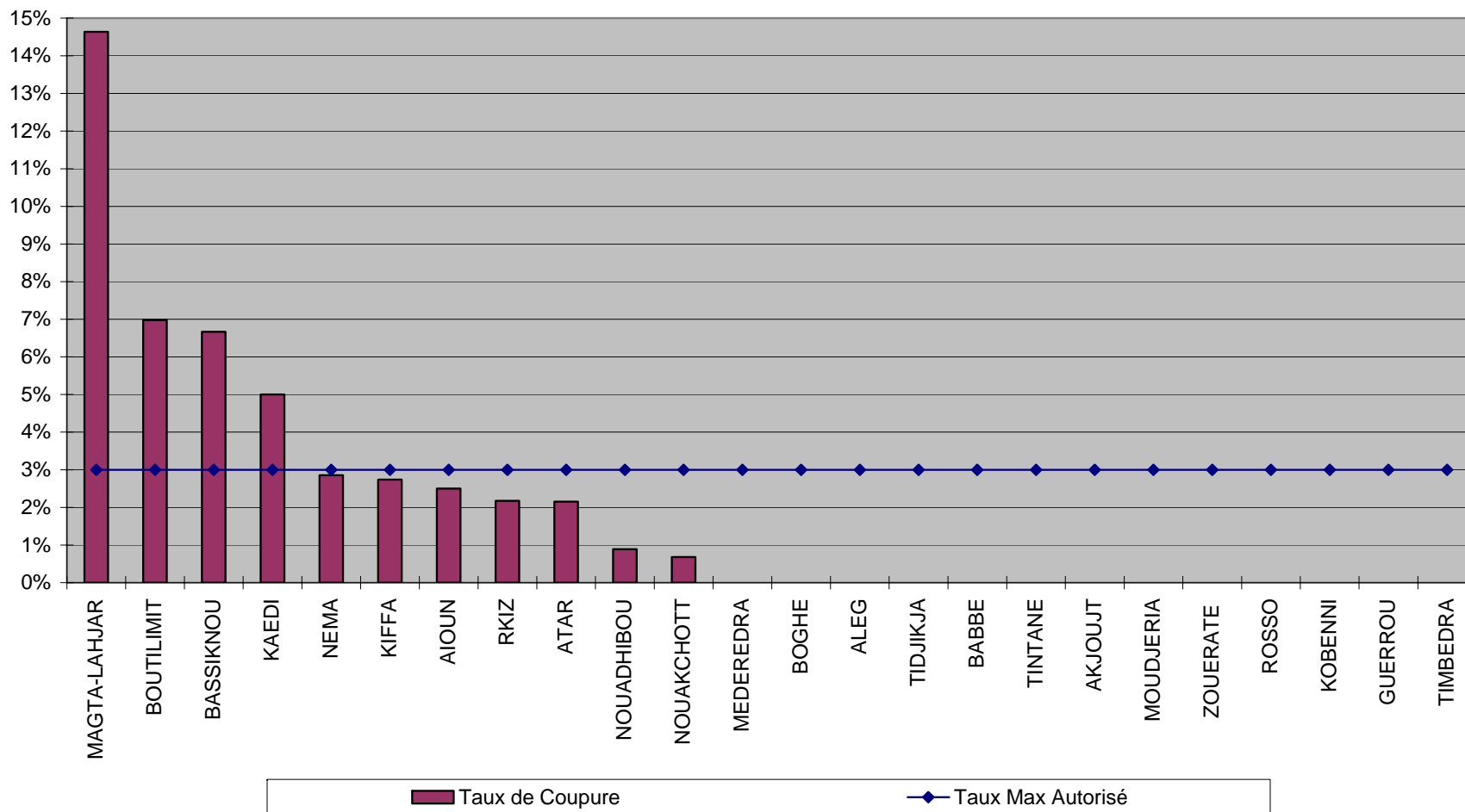
Taux de coupure d'appels (Mauritel)
