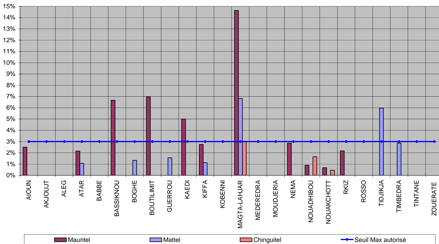
Taux de coupure d'appels pour les trois opérateurs
