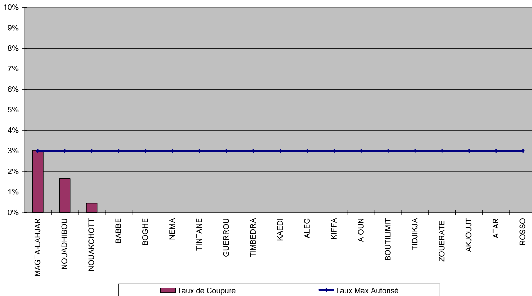
Taux de coupure d'appels (Chnguite)
