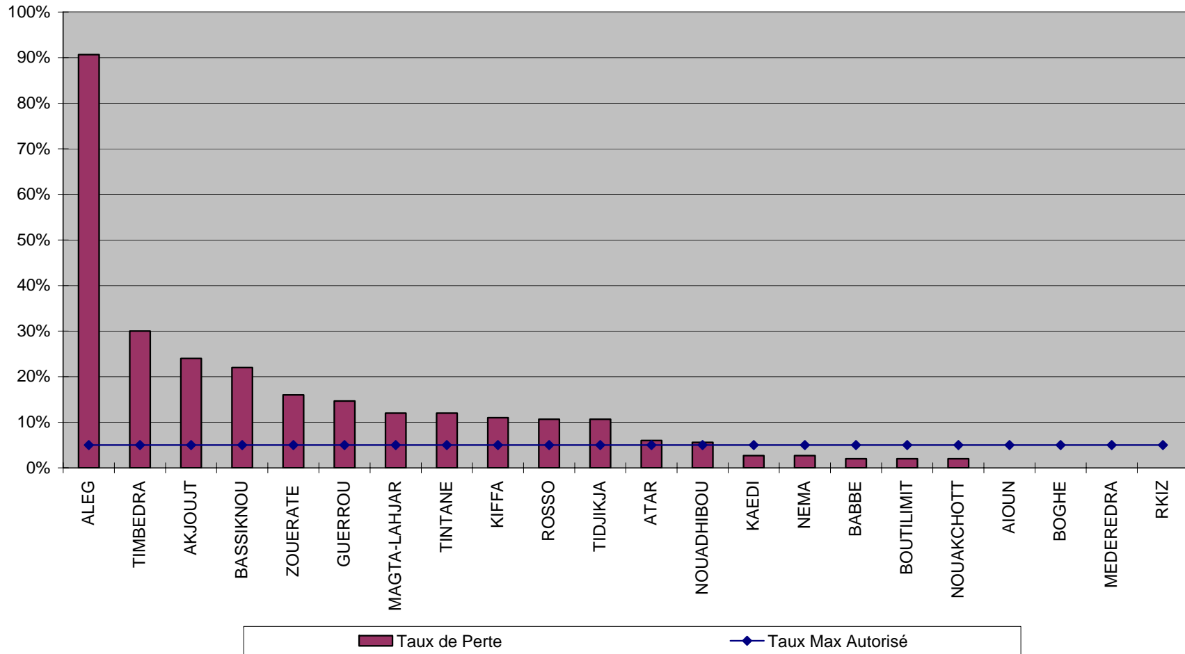
Taux de perte d'appels (Mattel)
